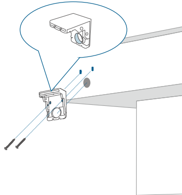
壁などに取り付ける場合
